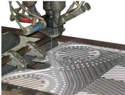
Aplicación de las juntas nuevas (pegadas o fijadas manualmente)
